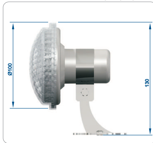
DIMENSÕES NA INSTALAÇÃO (mm)
